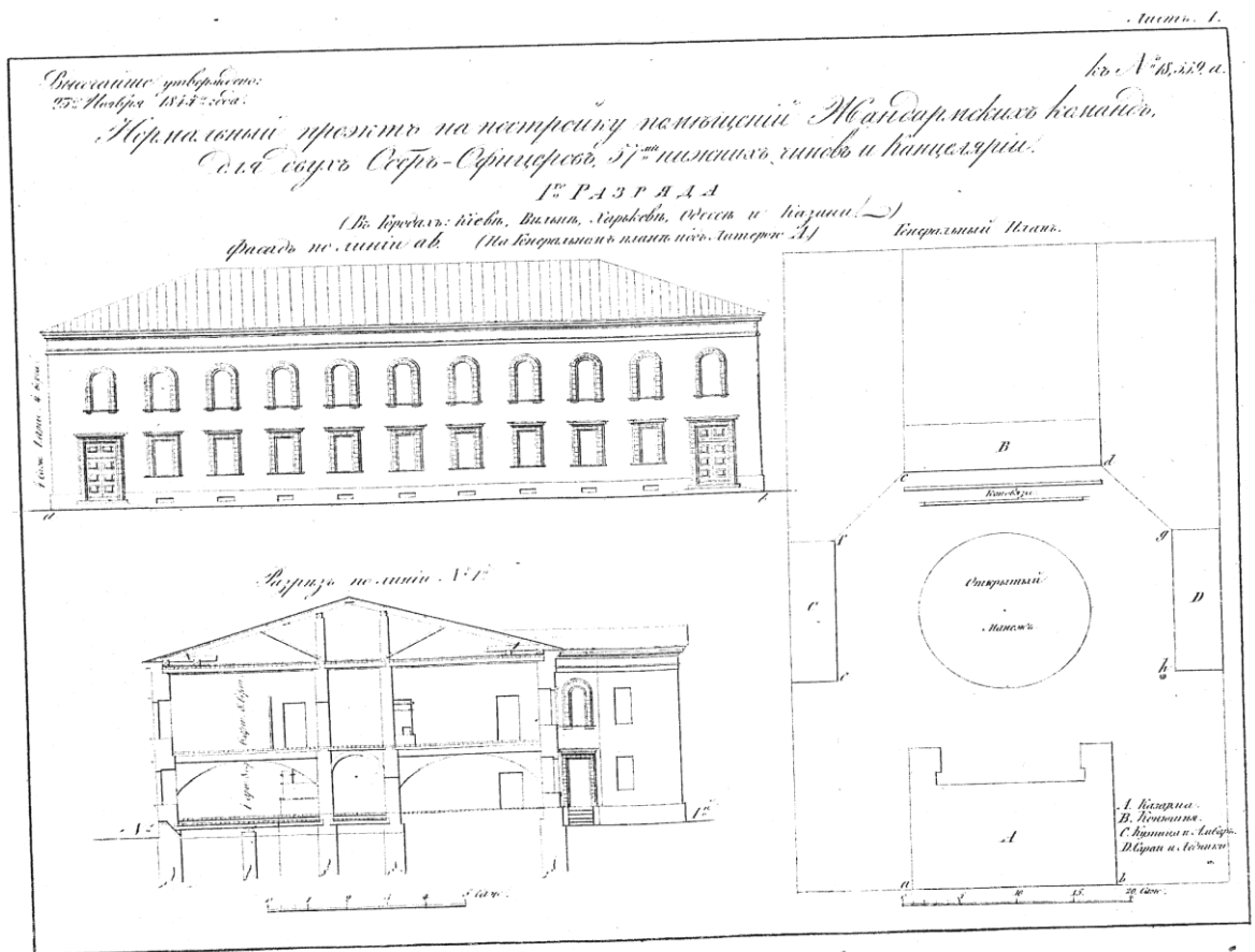
Чертежи ПСЗ. № 18559а от 25 декабря 1845 г.
